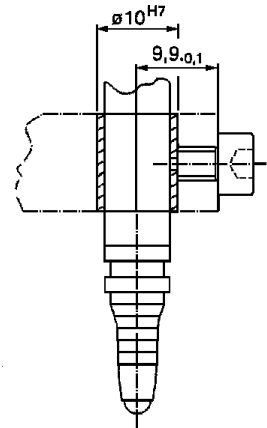
Einschraubvorschrift
