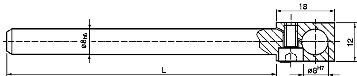
Klemmelement
