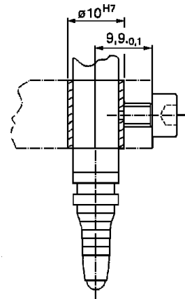
Einschraubvorschrift
