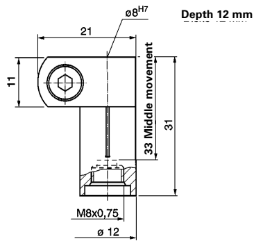
Article-No. 1124 01 (0°)
