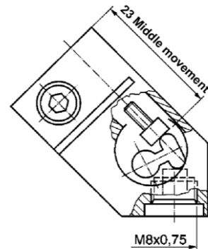
Article-No. 1124 03 (45°)
